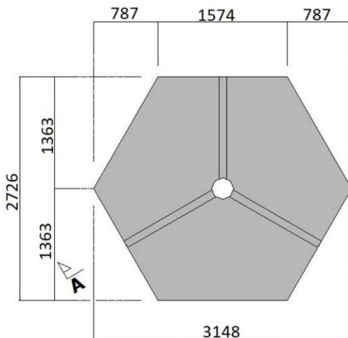
Grundriss der Fundamente
