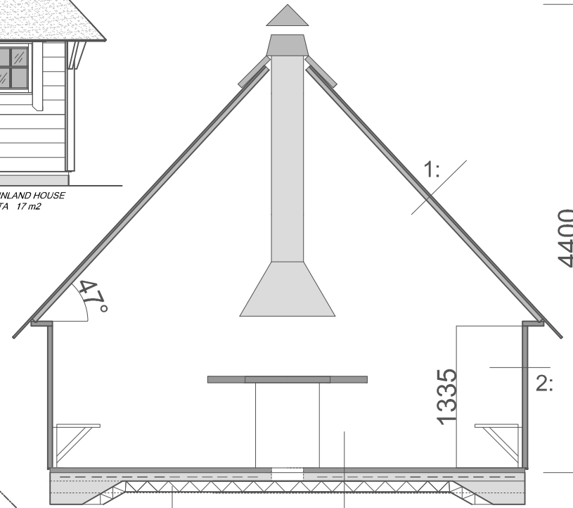
ARCTIC FINLAND HOUSE GRILLKOTA 17 m 2 Luftrohr für grill Ø 110 x 3
